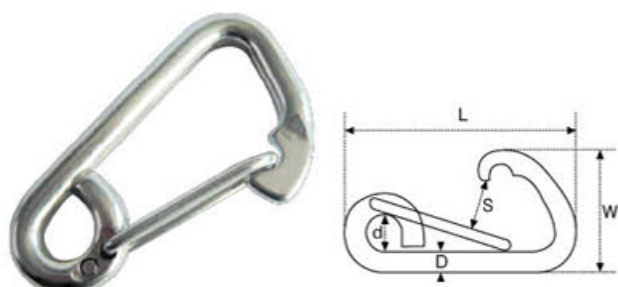
Delta Simple Snap Hook 平头简易弹簧钩
